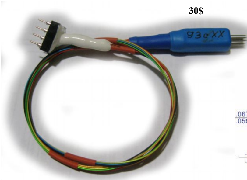
13. Щуп погопиновый SOT 23-6 93сXX, с DIP8 разъемом. Pogo pin test probe SOT 23-6 93сXX, with DIP8 plugs.
